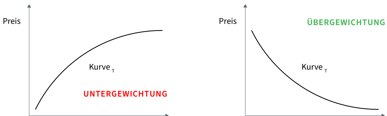
Abbildung 1: Querschnitts-Backwardation
