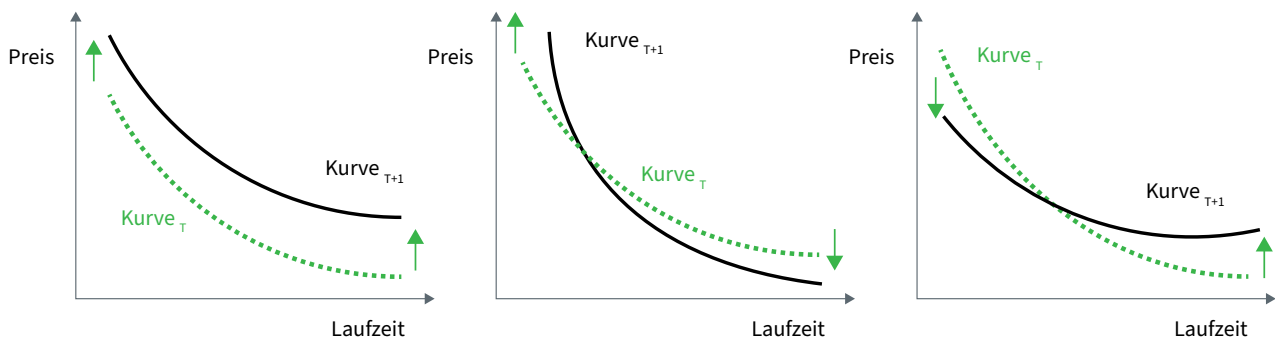
Abbildung 2: Steigungsdynamik
